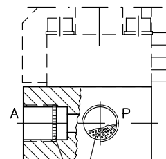
Elementi filtranti HFC secondo D 7235
